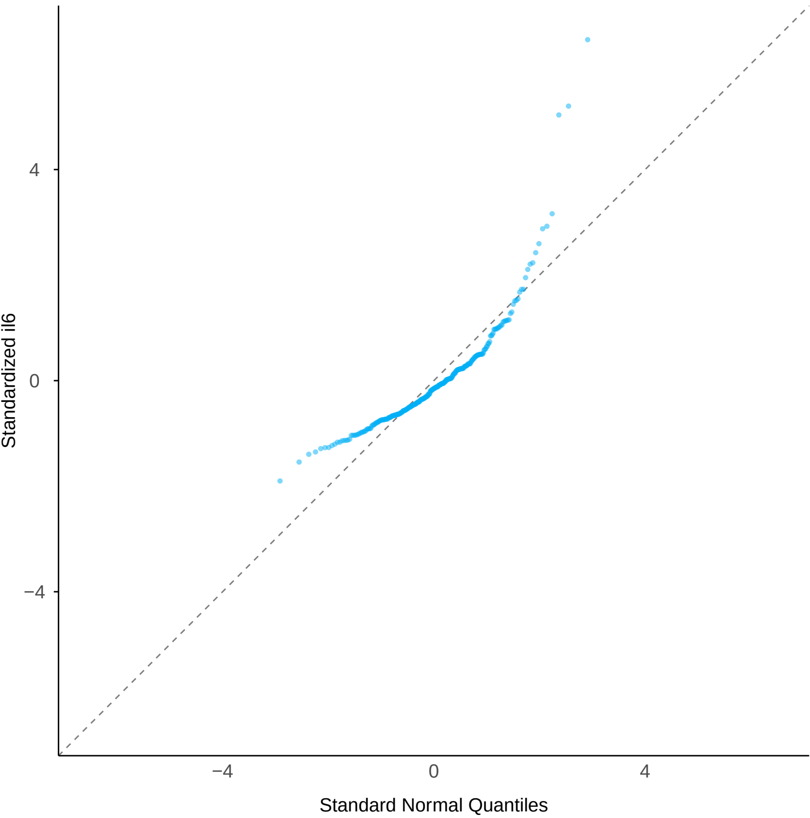
Normal Q-Q: il6
