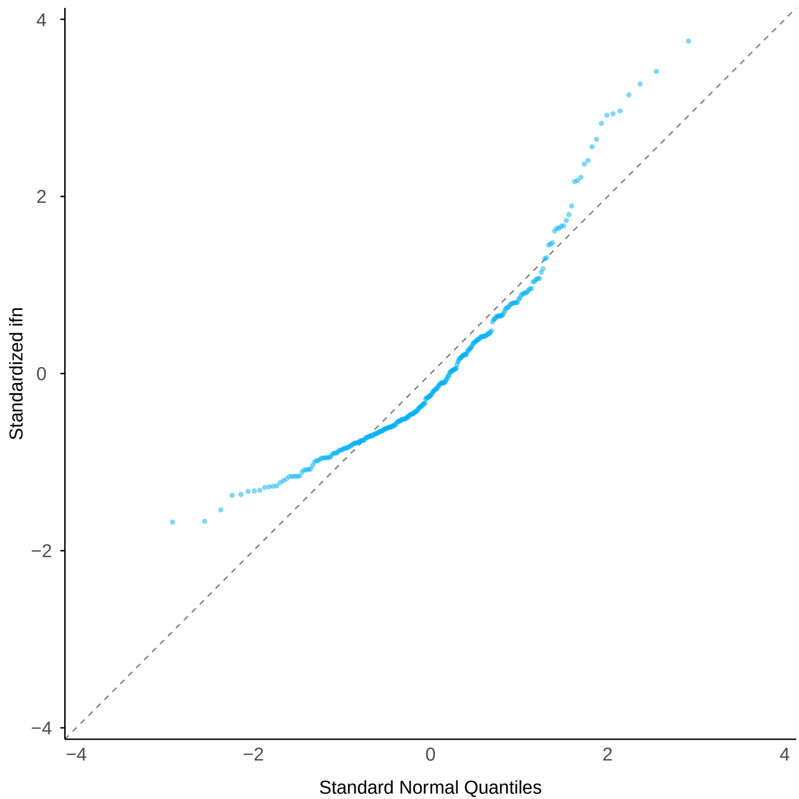
Normal Q-Q: ifn
